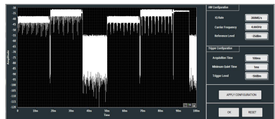
Мощносто-временная диаграмма и конфигурация триггера
